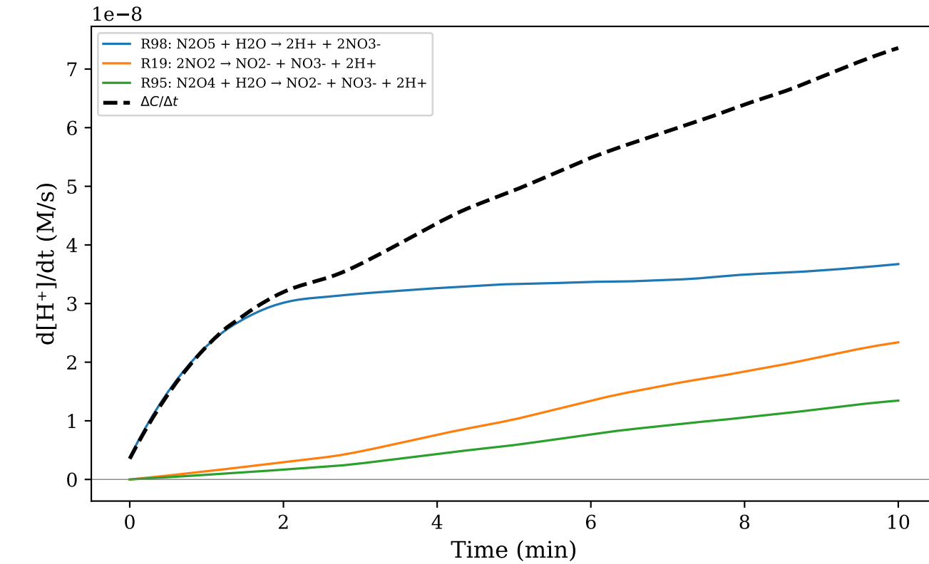
(d) H + [final=28.38 μM]
